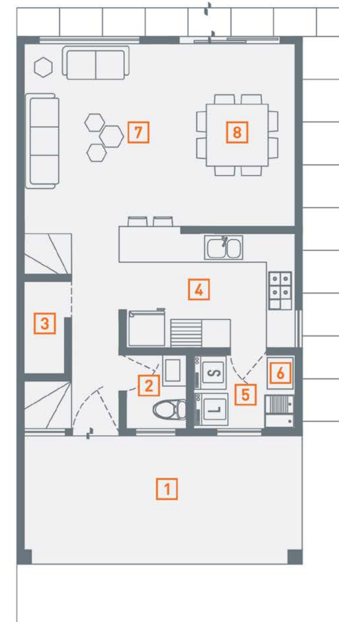
PLANTA BAJA
