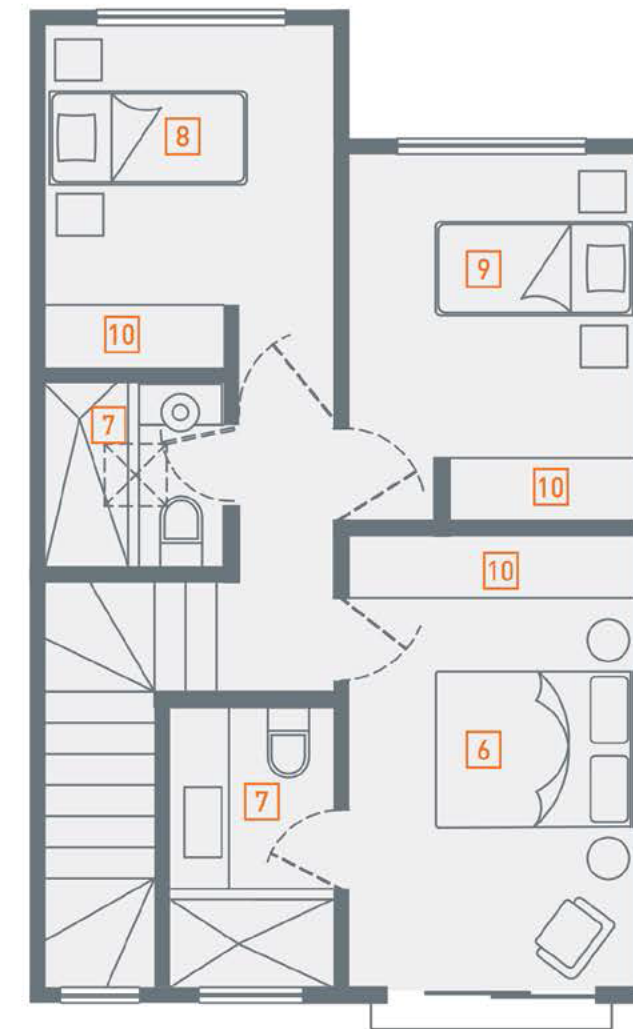
PLANTA ALTA
