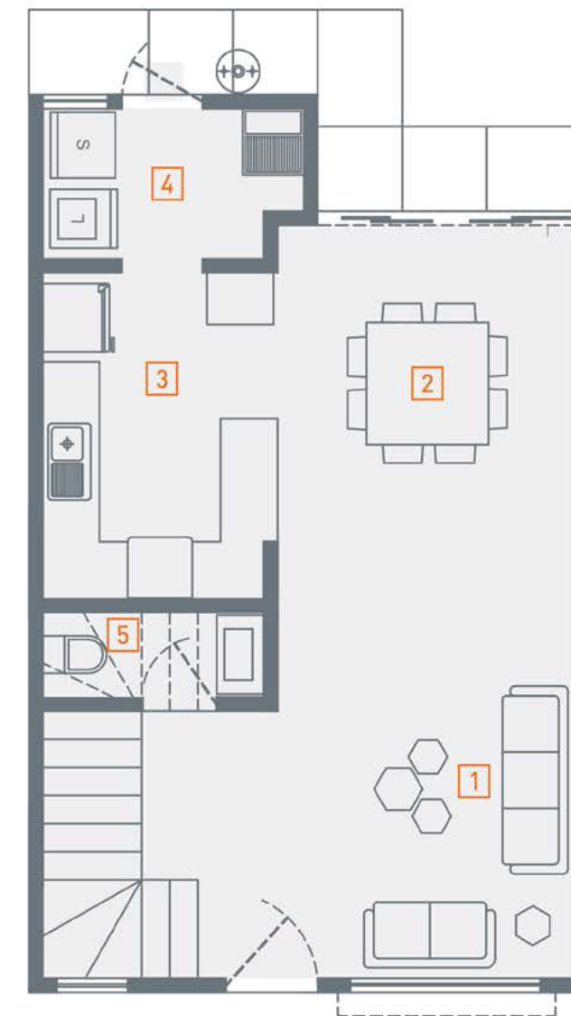
PLANTA BAJA
